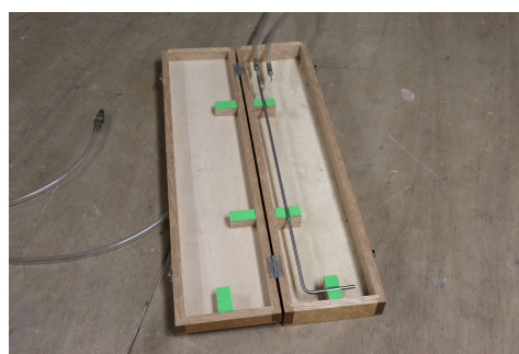
(b) ピトー管 (大阪公立大学所有)
