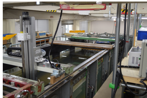
図 5: 回流水槽
